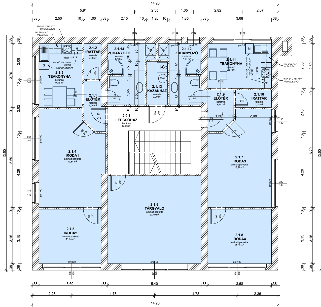
Mohács, Tompa Mihály utca 15. II. EMELET ALAPRAJZA M1:500
